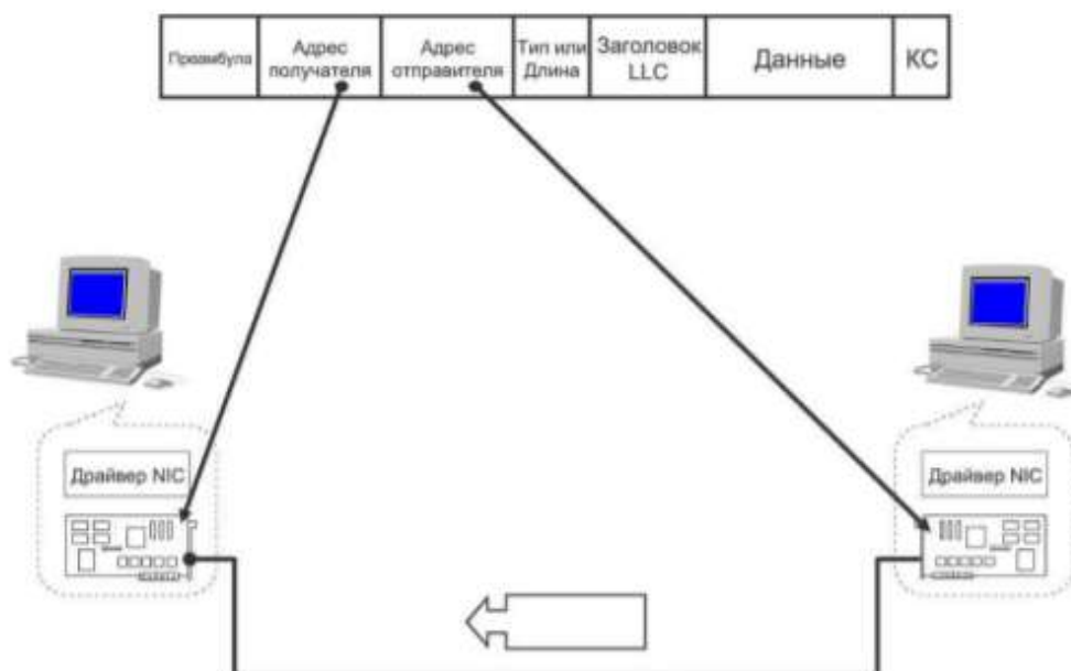
Рис. 2.3. Кадр Ethernet
